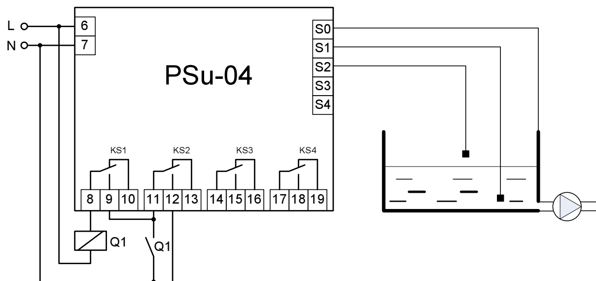
Rys 1. Sterowanie pracą pompy w zbiorniku przewodzącym. Górna sonda załącza, a dolna wyłącza.
