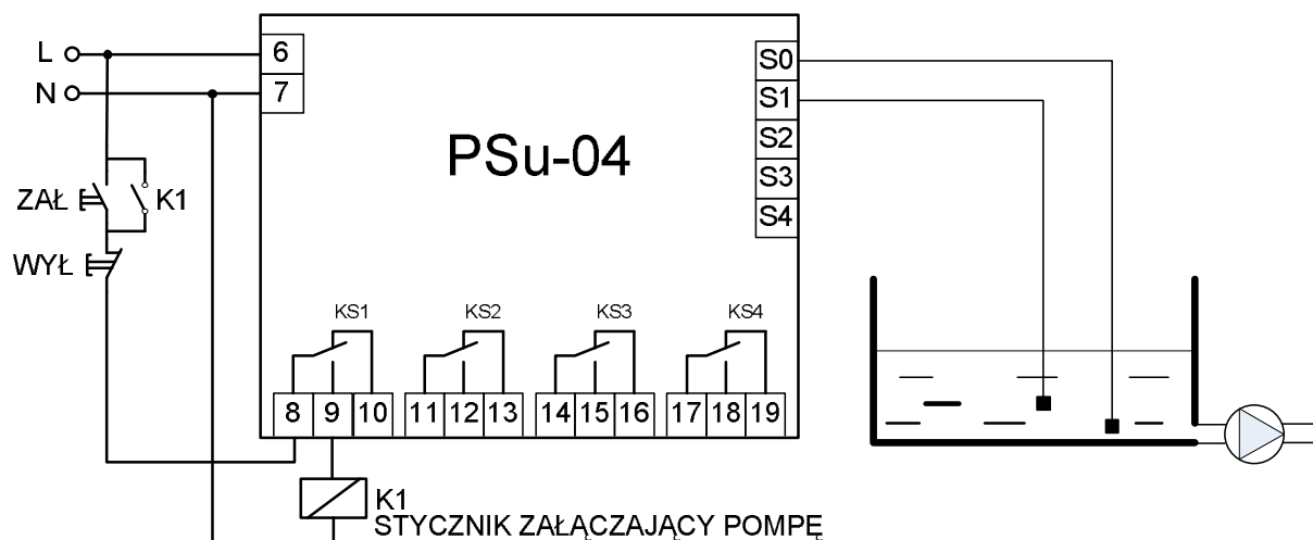
Rys 2. Układ sterowania pracą pompy opróżniającej zbiornik (nieprzewodzący) z wykorzystaniem PSu-04 do zabezpieczenia pompy przed suchobiegiem.
