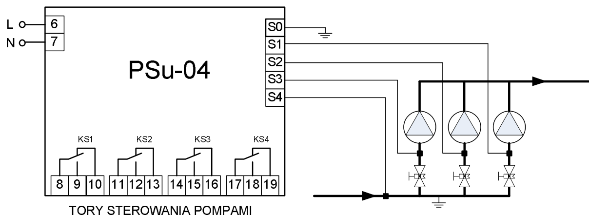
Rys 4. Układ indywidualnego oraz zbiorczego zabezpieczenia pomp przed suchobiegiem.
